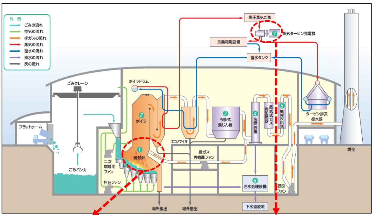
焼却炉（ストーカ）
