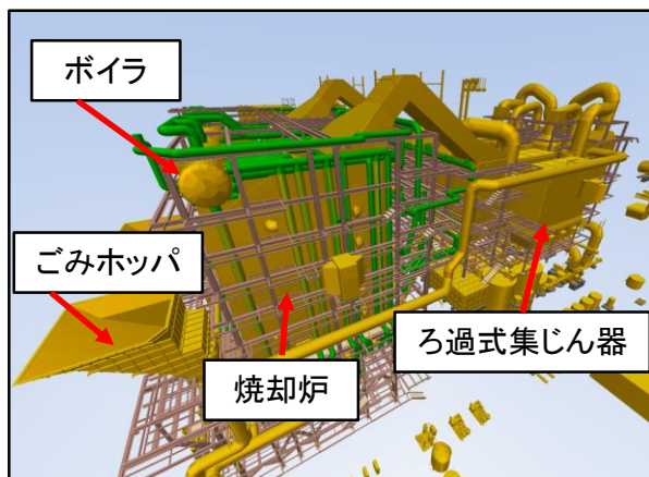
3次元図面の活用
