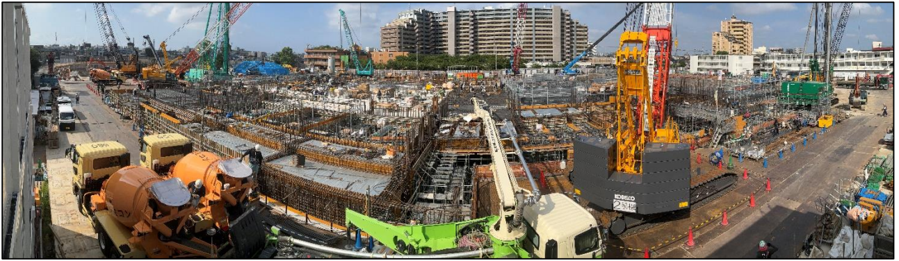
8月 工場棟地下1階床コンクリート工事を終え、地下1階壁・柱の工事を進めています。
