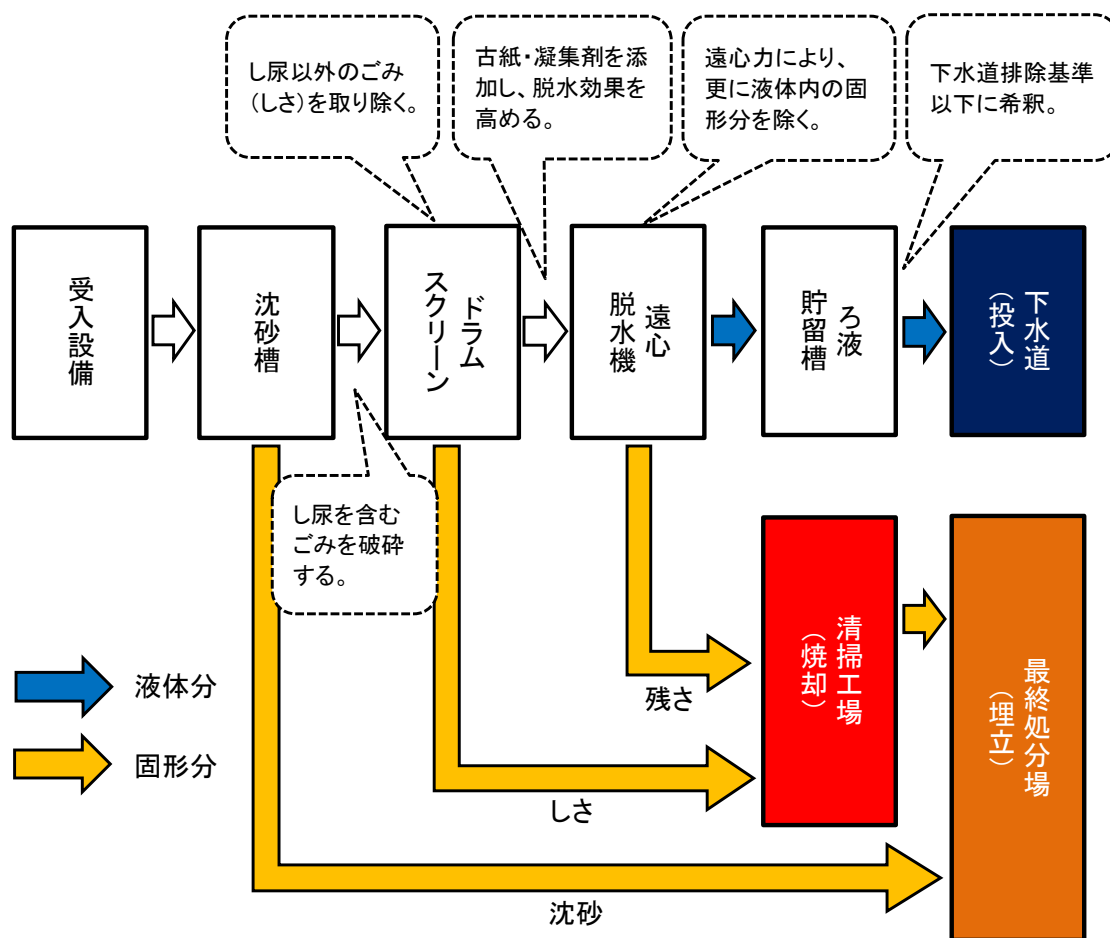
図－1 品川清掃作業所におけるし尿の下水道投入までの流れ
