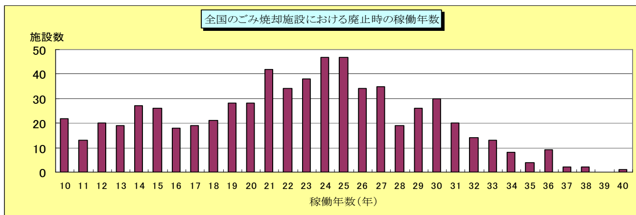
図－25 全国のごみ焼却施設における廃止時の稼働年数
