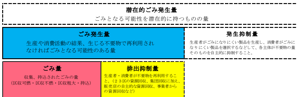
図-1-10 ごみ量の概念
