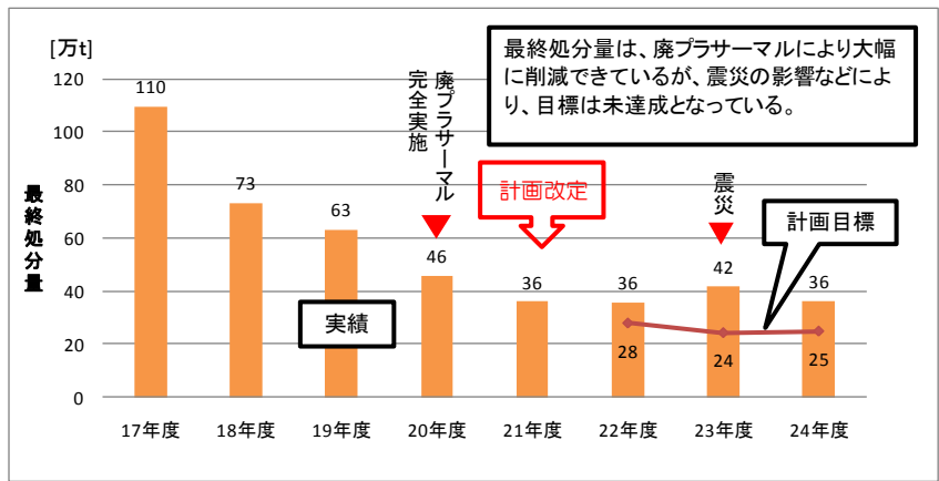
図－2－10 最終処分量の推移
