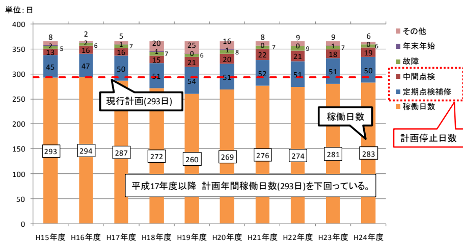
図-2-20 清掃工場の稼働実績（1炉当たり）
