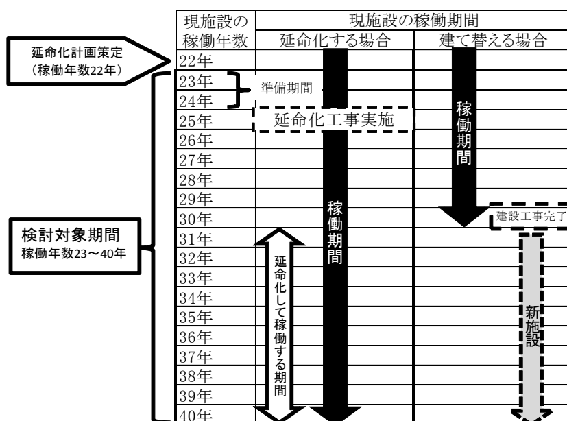
図-1-13 検討対象期間の設定
