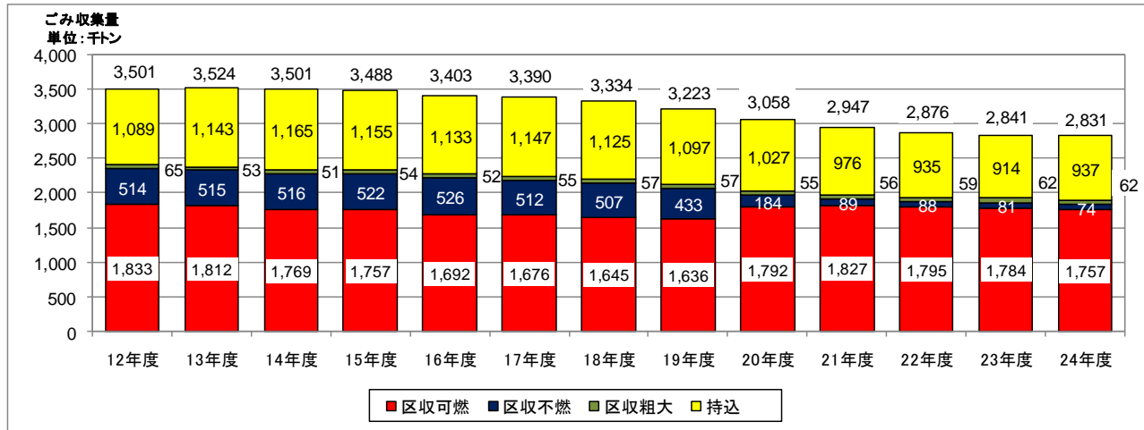
図-1-4 ごみ収集量の推移
