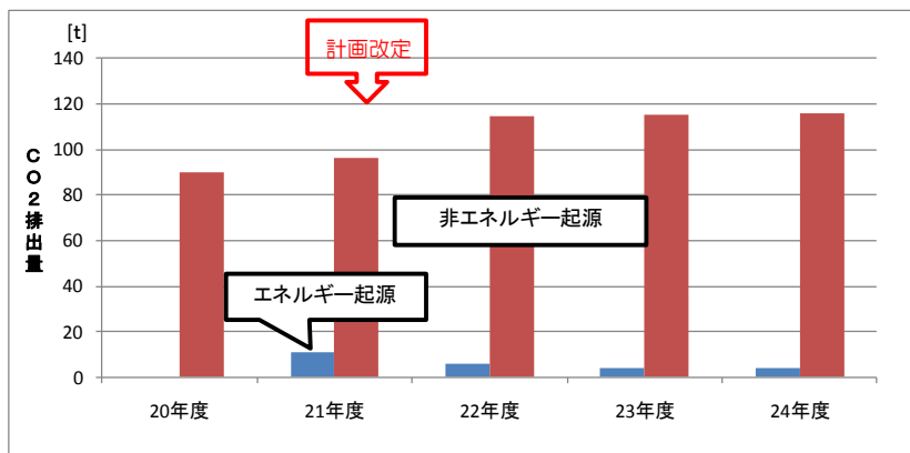
図-2-6 温対法によるCO 2 排出量
