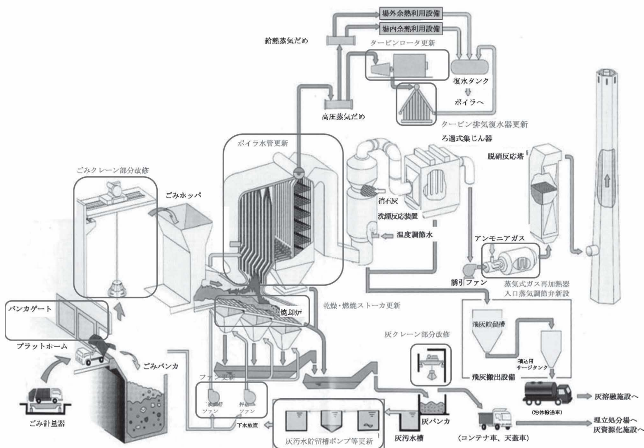
図Ⅲ－15 千歳清掃工場延命化工事の主な項目
