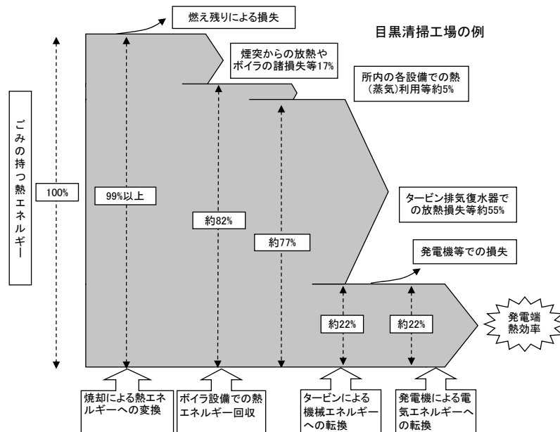
図Ⅲ－３ 清掃工場における熱効率イメージ図
