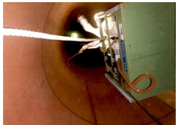
清掃の様子 煙突内壁をゴンドラに乗って 清掃中(下からの撮影)
