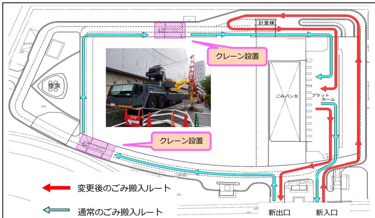
港清掃工場 平面図
