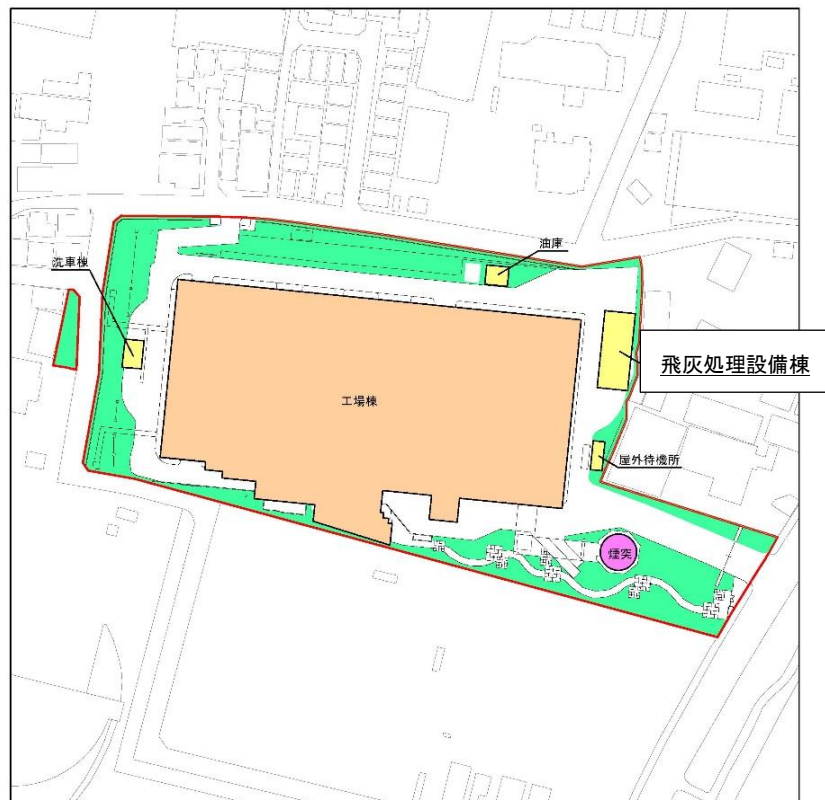
図ー1 施設配置イメージ図
